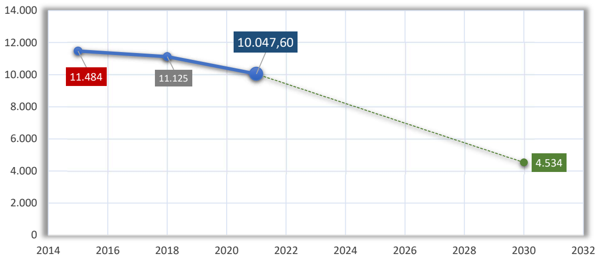
I.13.2.1 Inventario de Emisiones de GEIs de la ciudad de Madrid. Kt CO2 equivalente
